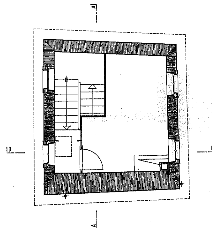
ETAGE 2
